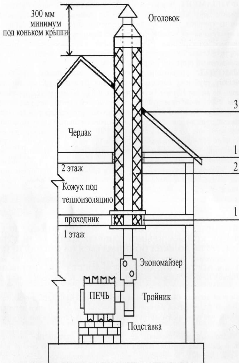
УСТАНОВКА ПЕЧИ С МЕТАЛЛИЧЕСКИМ ДЫМОХОДОМ ВНУТРИ 2-ЭТАЖНОГО ДОМА
